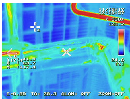
(ب) تصویر ترموگرافی خطوط انتقال
