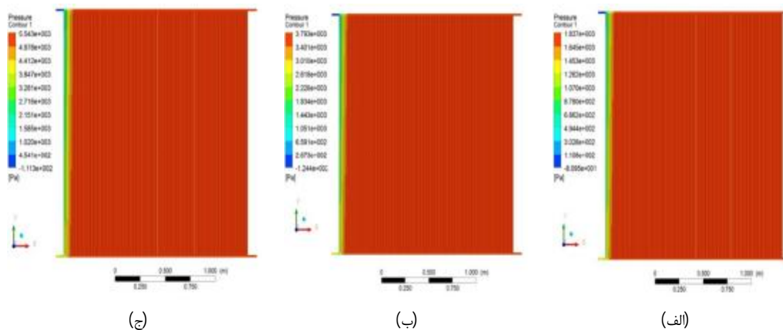
شکل ۷- کانتور فشار برای الف) دبی 0.06 لیتر بر ثانیه، ب) دبی 0.1 لیتر بر ثانیه، ج) برای دبی 0.14 لیتر بر ثانیه
