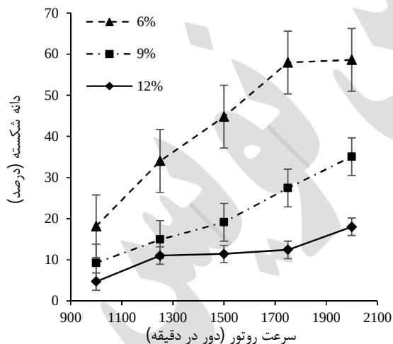
شکل ۶- تغییرات درصد دانه شکسته رقم هاشمی با سرعت دورانی روتور در سطوح محتوای رطوبتی متفاوت
