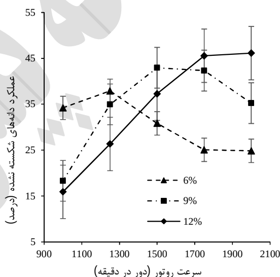
شکل ۷- تغییرات درصد عملکرد دانه‌های شکسته نشده رقم هاشمی با سرعت دورانی محور در سطوح محتوای رطوبتی متفاوت
