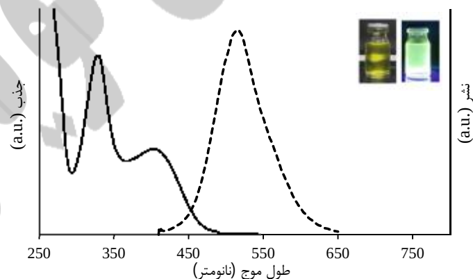
شکل ۵- منحنی جذب (آبی) و نشر (سبز) نقاط کوانتومی کربن. تصویر داخلی مربوط به محلول حاوی نقاط کوانتومی کربن در زیر نور محیط و نور فرابنفش را نشان می‌دهد.
