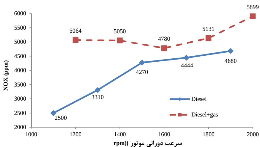
شکل ۸- میزان \text{NO}_x تولیدی موتور در هر دو سامانه
