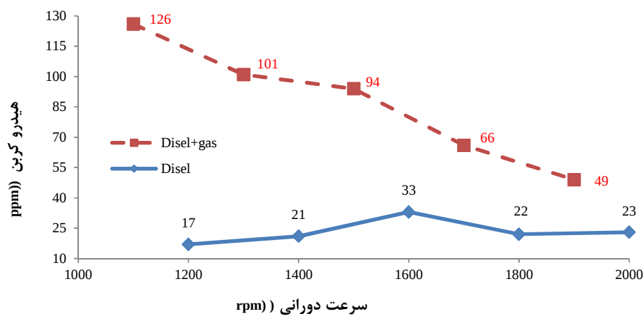
شکل ۷- میزان آلاینده‌گی هیدروکربن
