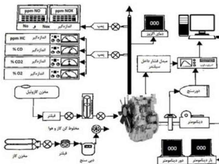
شکل ۱- طرح‌واره اجزاء آزمون‌های عملکردی و آلایندگی موتور مورد نظر
