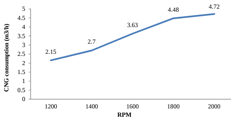
شکل ۴- میزان مصرف سوخت گاز طبیعی فشرده برای موتور با سوخت ترکیبی
