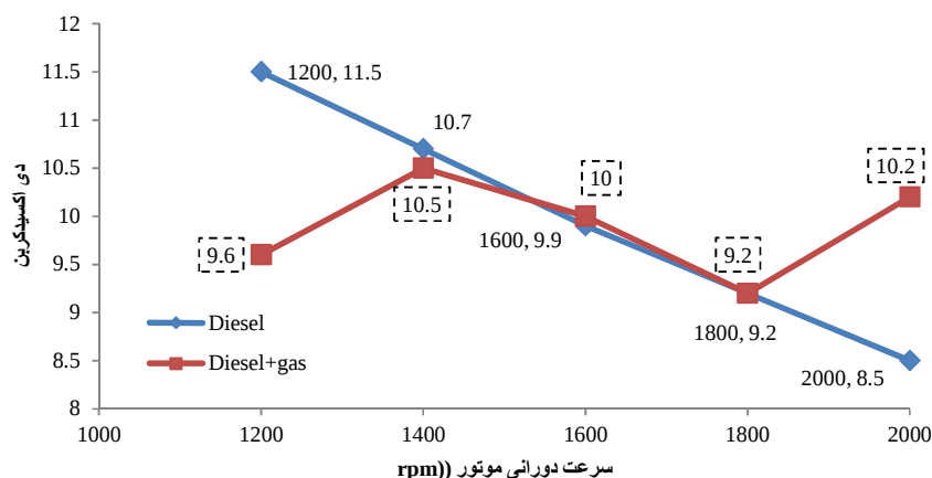
شکل ۹- میزان دی اکسید کربن تولیدی موتور در حالت دیزل و ترکیبی
