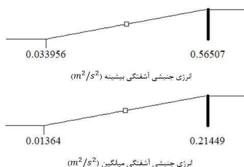
شکل ۴- شرایط مرزی و نقطه بهینه در روش سطح پاسخ
